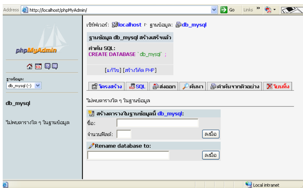
รูปที่ 4 ตัวอย่างผลการสร้าง Database ใหม่
