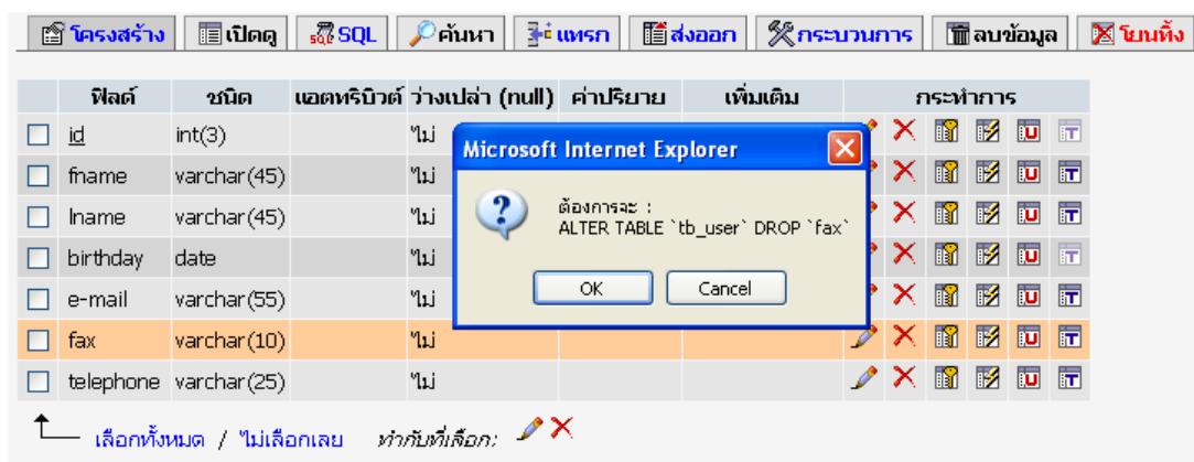
รูปที่ 13 หน้าต่างการยืนยันลบฟิลด์ออกจากตาราง
