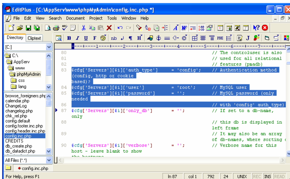
รูปที่ 2 กำหนด User และ Password เข้าใช้งาน
